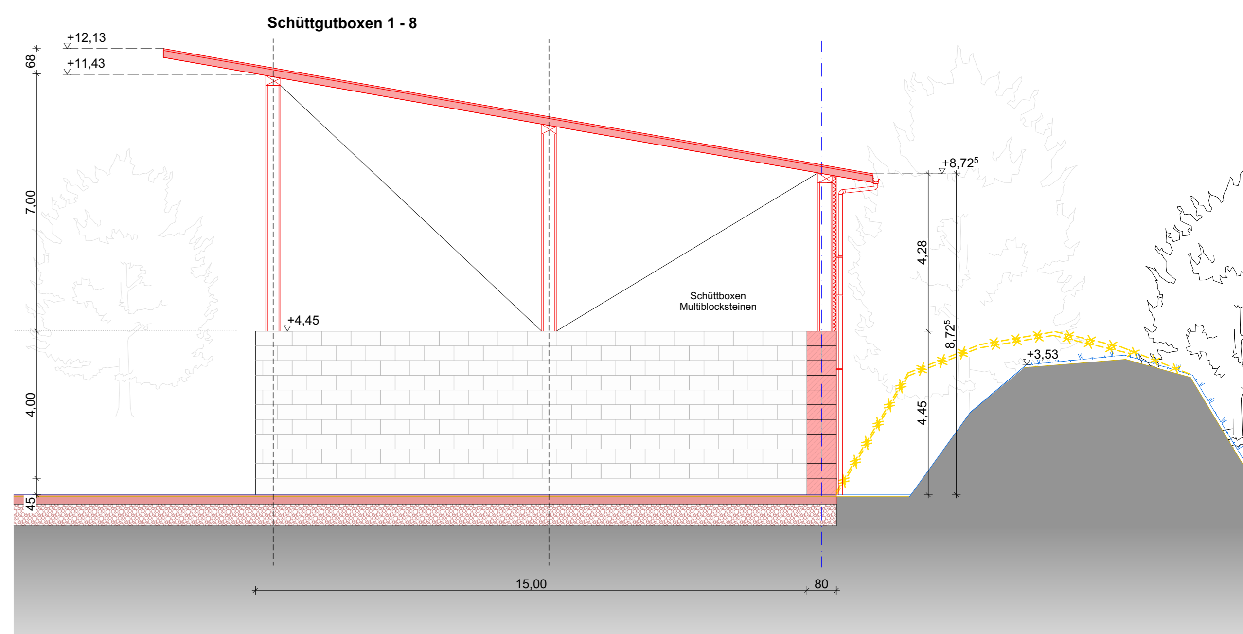
SCHNITT 1 - 1
