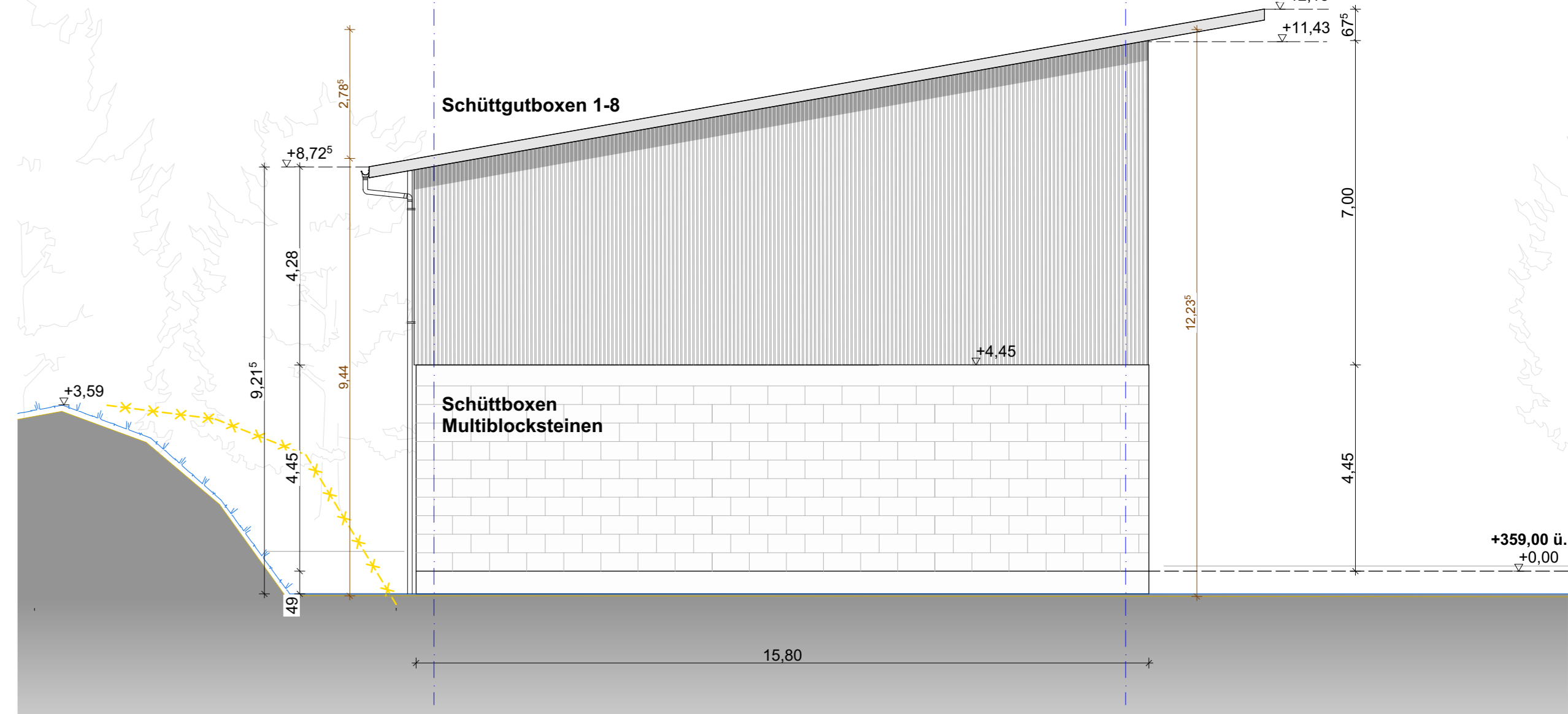
SCHNITT 2 - 2
